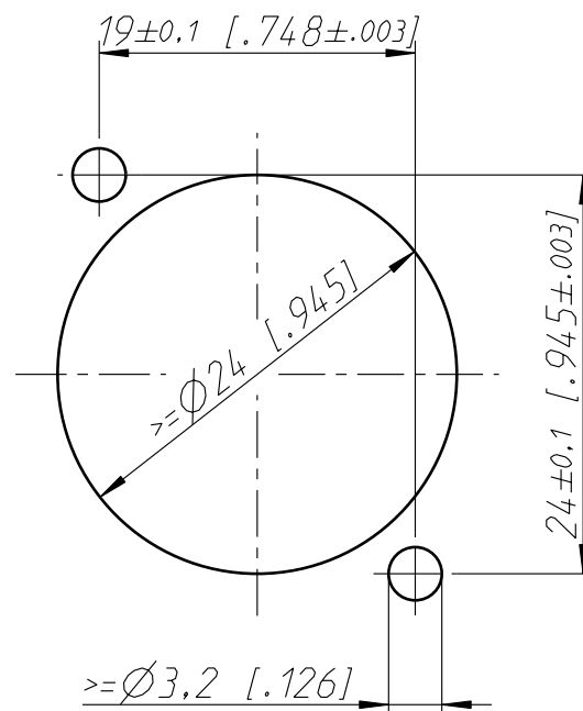
Frontplattenausschnitt (Rückseite) Panel cutout (rear side)
