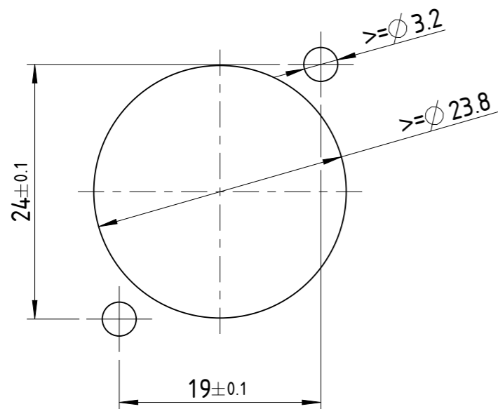
Frontplattenausschnitt (Rückseite) Panel cutout (rear side)
