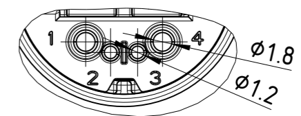
Lötkontakte Rückseite Soldering contacts rear side
