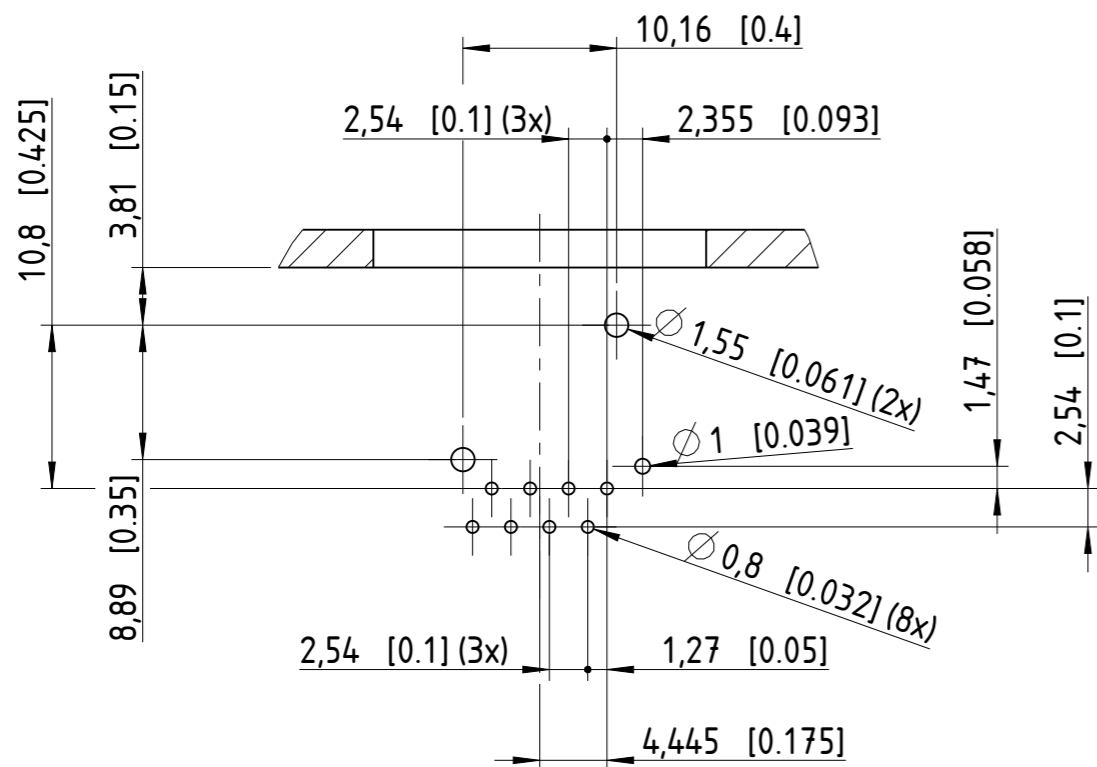
2:1 Print Bohrplan Bestückungsseite PCB-Layout (component side)
