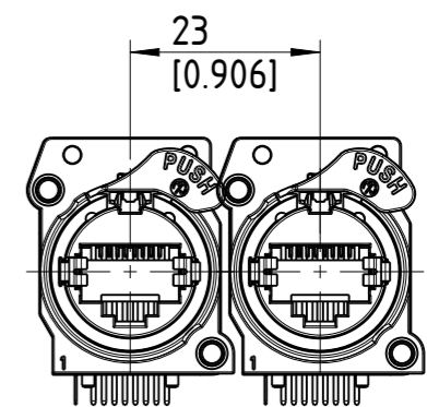
1:1 min. Einbauabstand min. assembling distance
