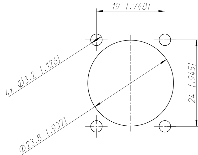
Frontplattenausschnitt panel cut out
