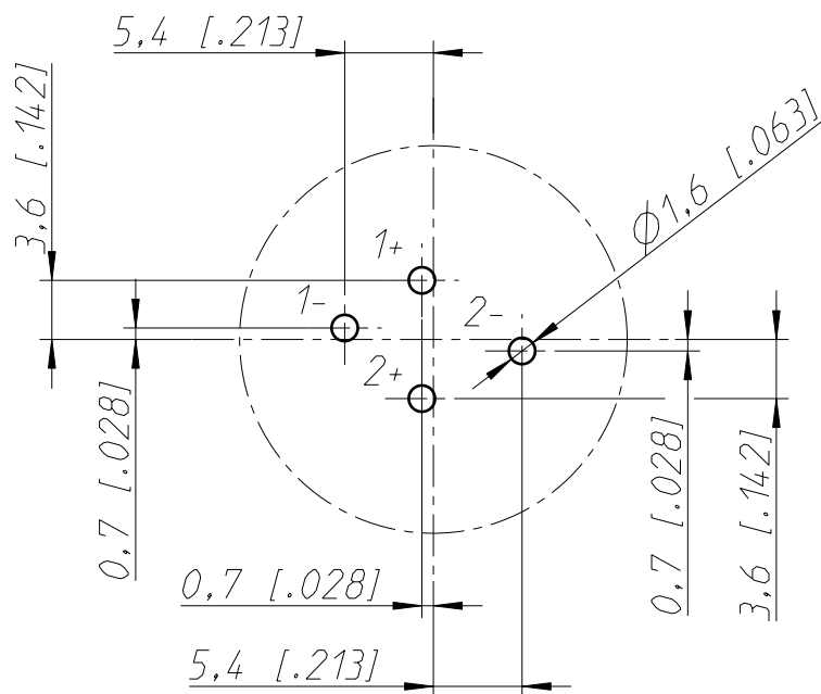
Leiterplatten Bohrplan Bestückungsseite PCB-Layout (component side) Toleranz ±0.05 [0.002]
